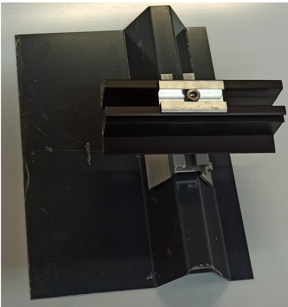
Modèle Opti'Roof
