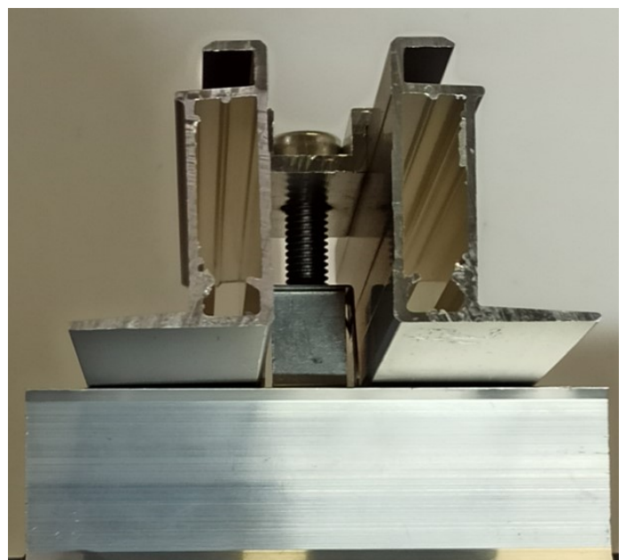
TERRAGRIF PL0.5*20*41
